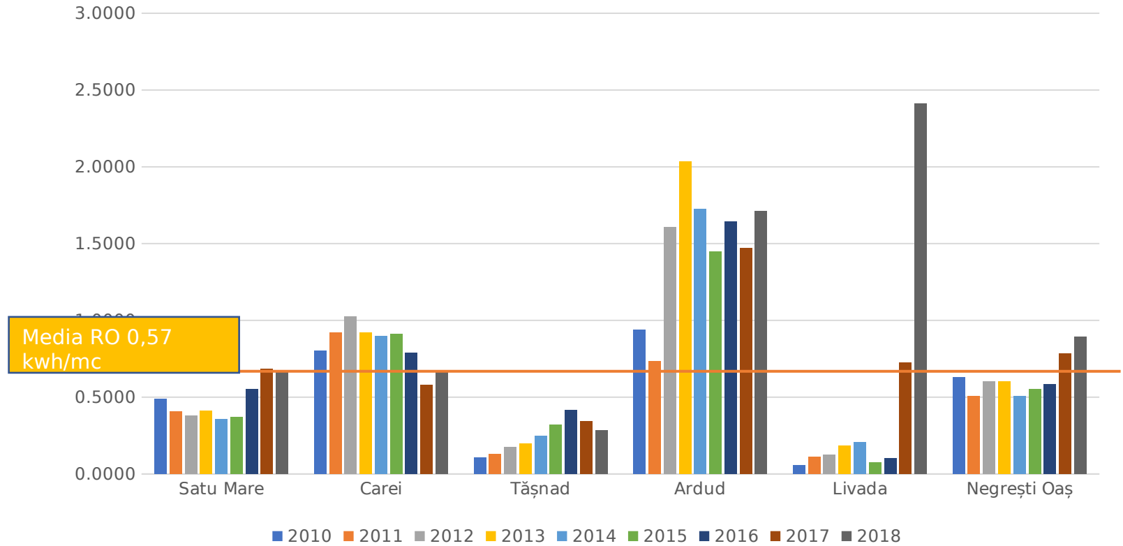
CONSUMUL DE ENERGIE PE M3 APĂ UZATĂ kWh/mc
