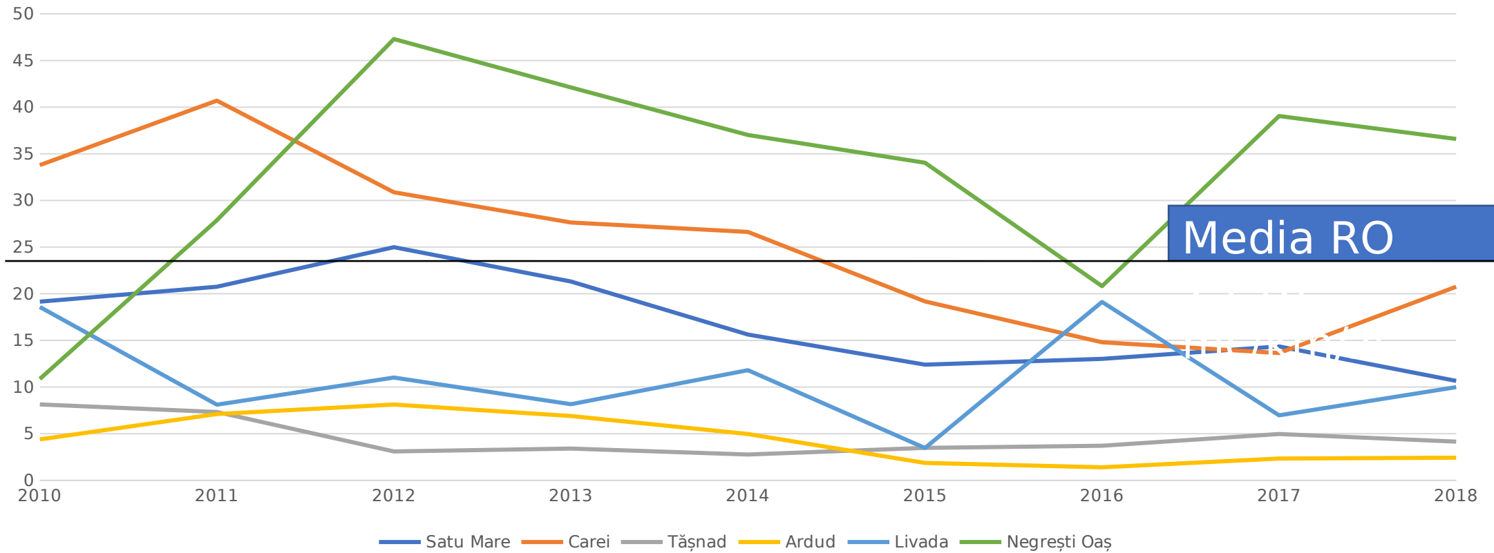
PIERDERI REALE LA NIVELUL REȚELEI DE APĂ m3/km/zi
